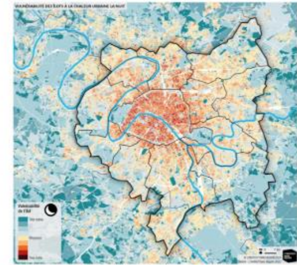
Figure 15 : Zones de la Métropole du Grand Paris vulnérables, la nuit, à l'effet d'îlot de chaleur urbain. Source : IFR 2024.
