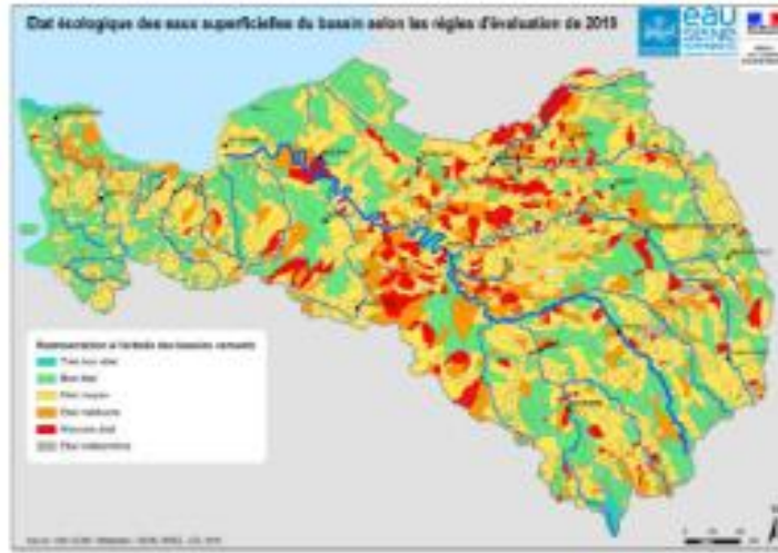
Figure 18 : Etat écologique des eaux superficielles du bassin de la Seine. Agence de l'Eau Seine-Normandie, 2015.
