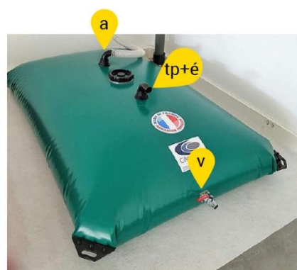
Citerne souple de 50 à 400 m³
